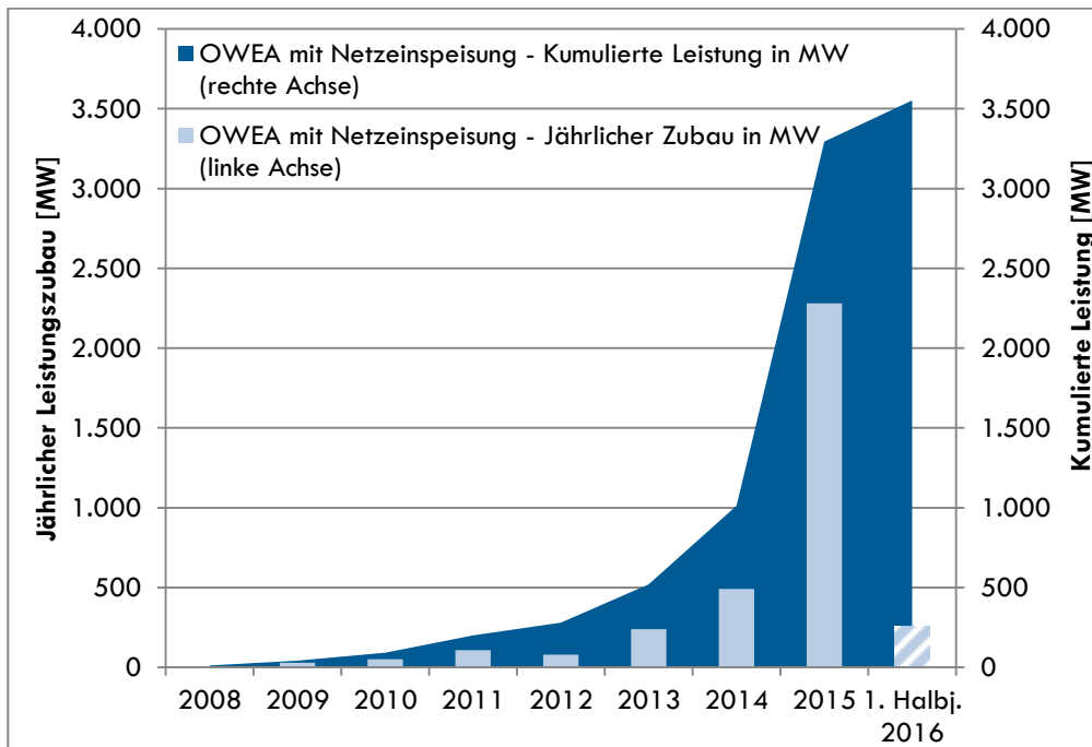
Abbildung 1: Entwicklung der Offshore-Windenergie in Deutschland (Kapazität der OWEA mit Netzeinspeisung), Stand 30.06.2016
